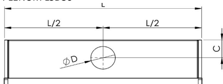
PLENUM LSD30
