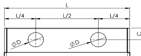
PLENUM LSD50
