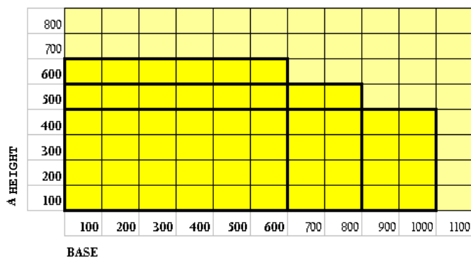
Serranda di taratura a contrasto: dimensioni realizzabili in soluzione unica
