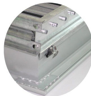
Serranda di taratura a contrasto: dettagli clips di fissaggio brevettata
