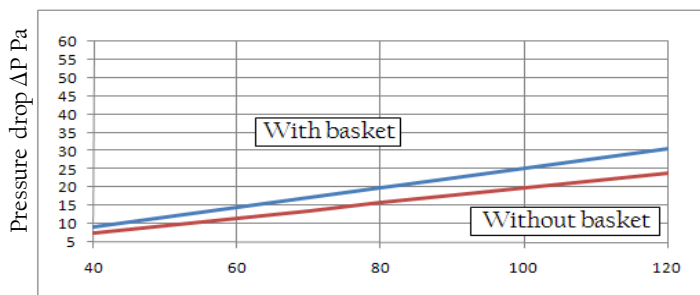
TE-KP160 Air flow m³/h
