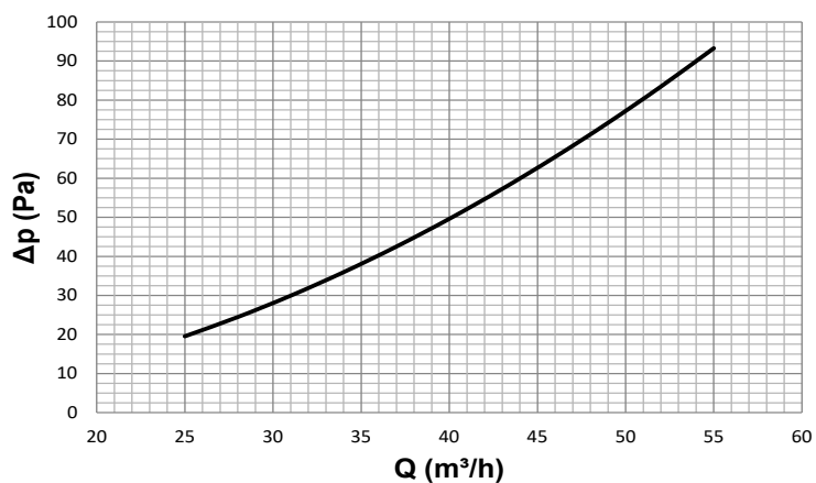
KV-40 Perdita di carico
