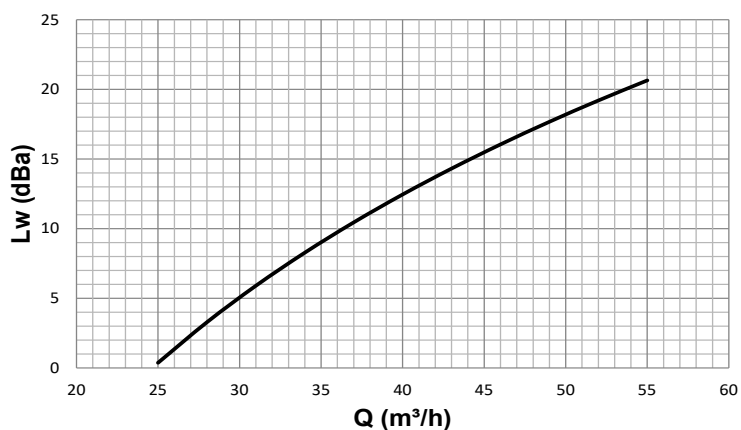
KV-40 Potenza sonora
